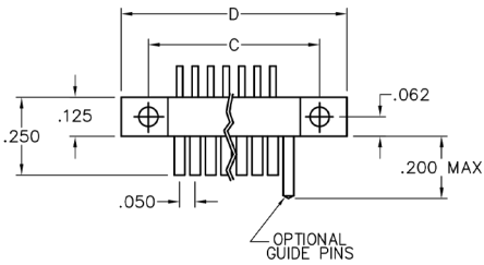
Receptacle
